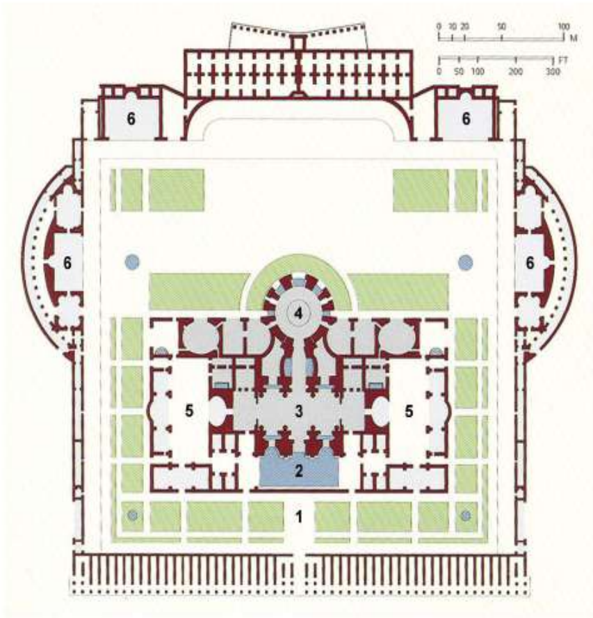
Figura 2 – Planta geral dos Balneários de Caracala, em Roma, 212-216 d.C., in Henri Stierlin, O Império Romano. Dos Etruscos ao Declínio do Império Romano , Taschen, 1999
